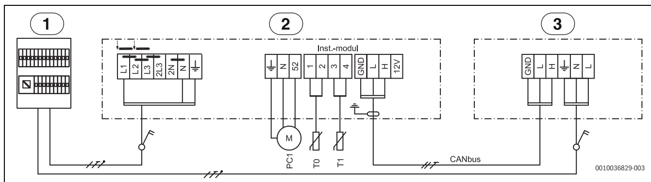
40. ábra 5,85 kW 230 V~os kapcsolási rajza
