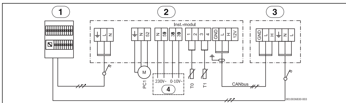
41. ábra 5,85 kW 3 N~es kapcsolási rajza
