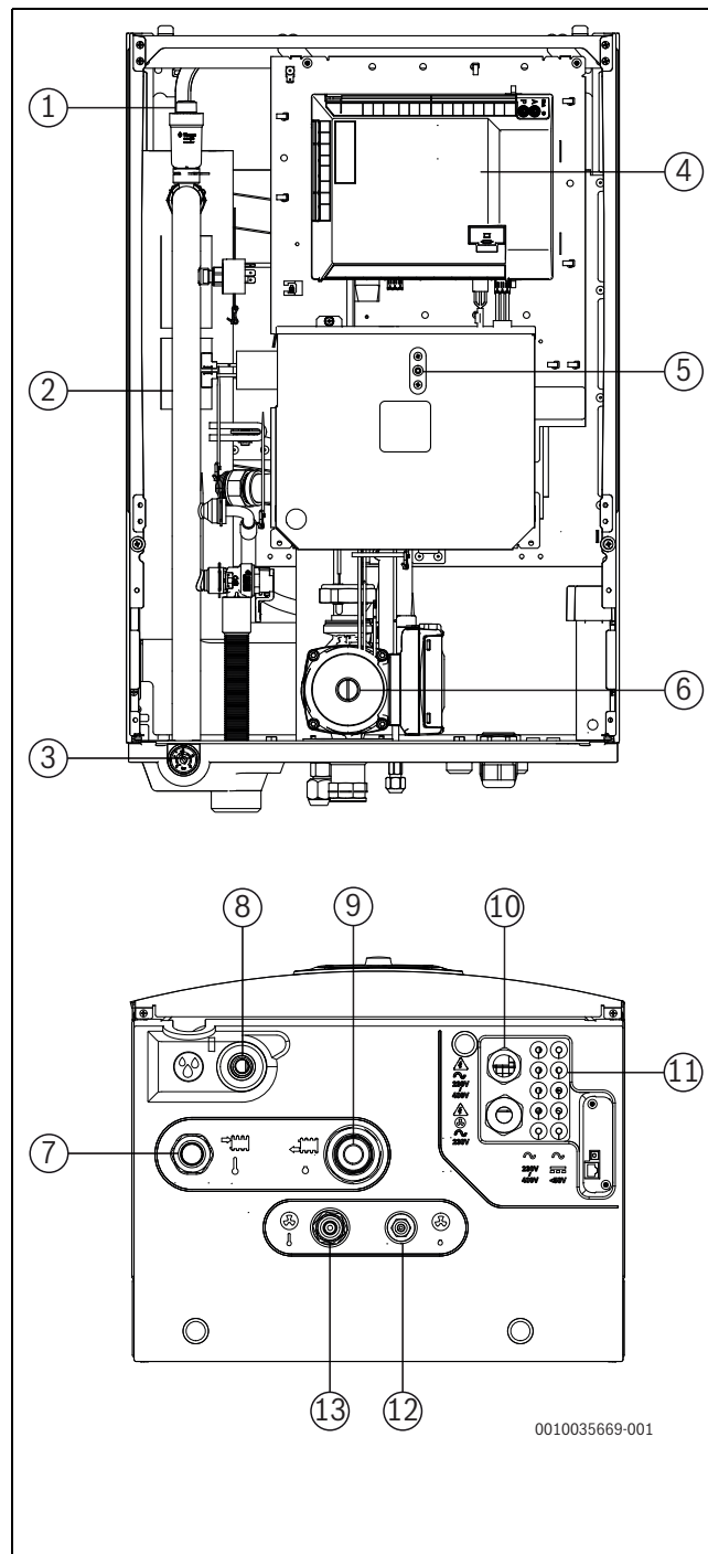
3. ábra Elektromos fűtésegységgel rendelkező beltéri egység alkatrészei és csővezeték-csatlakozásai (csepegtetőtálcával)
