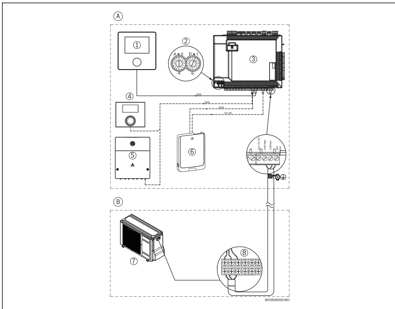
39. ábra CAN-BUS és EMS csatlakozó
