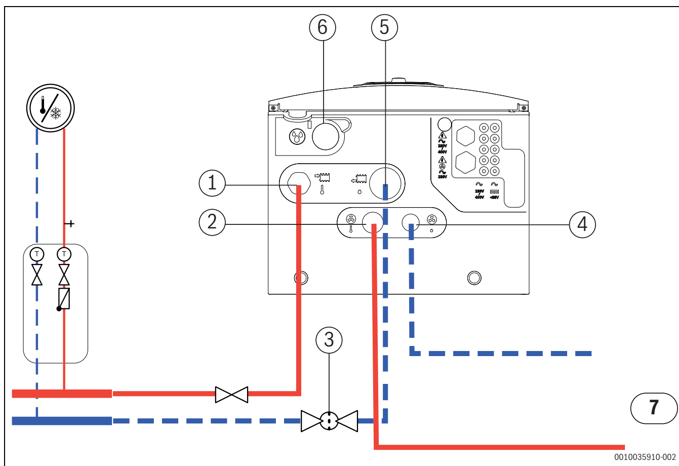
8. ábra Beépített elektromos fűtésrsegítéssel bíró beltéri egység csatlakoztatása kültéri egységhez és fűtési rendszerhez.
