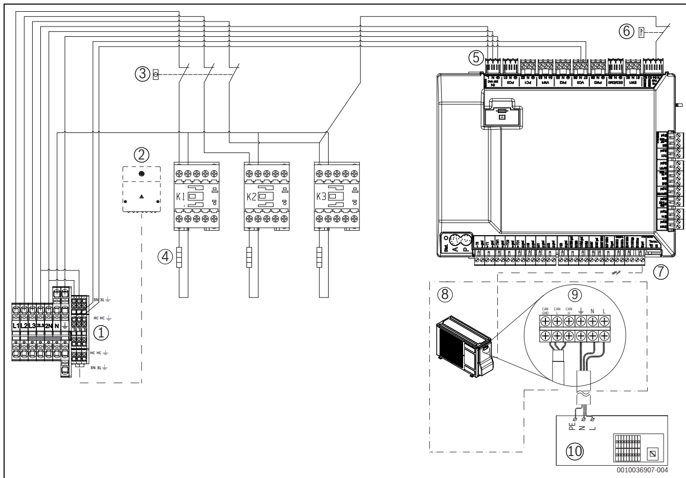
42. ábra 400 V 3 N~ beltéri egység 230 V~ kültéri egységgel
